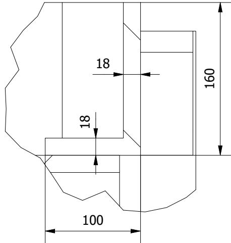
H ( 1 : 4 )
