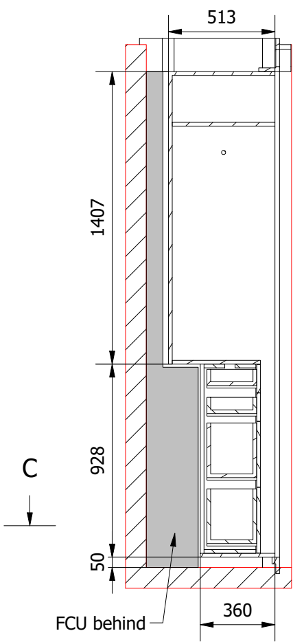
A-A ( 1 : 25 )
