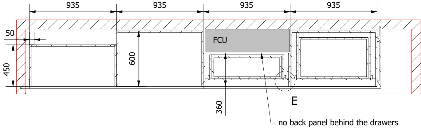
C-C ( 1 : 25 )
