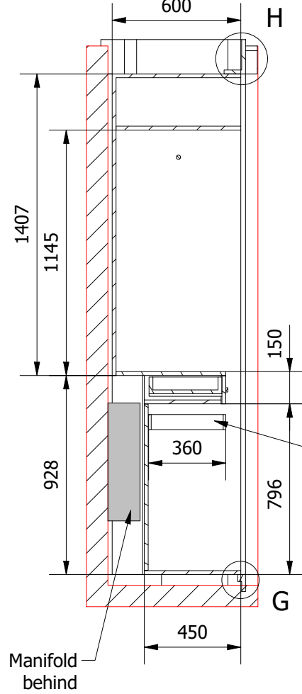
B-B ( 1 : 25 )
