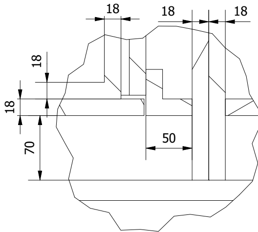
E ( 1 : 4 )
